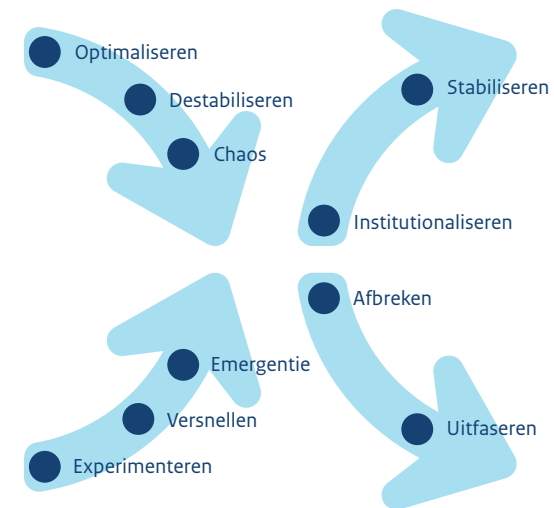
Figuur 1. De X-curve van transitie. De X-curve is een concept of raamwerk waarin onderscheid wordt gemaakt tussen patronen van opbouw en afbouw die elkaar versterken of tegenwerken. Het figuur is afkomstig van het rapport sturing in transitie van DRIFT (31).
